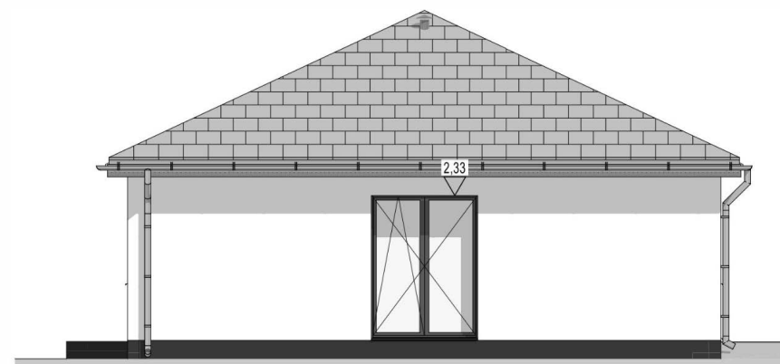
4 Elewacja BOCZNA 1:100
