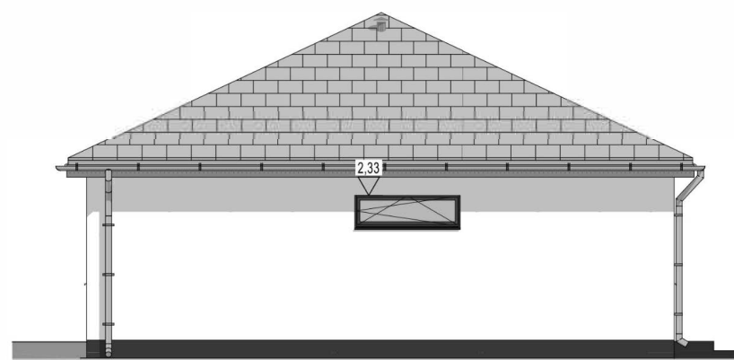
2 Elewacja BOCZNA 1:100
