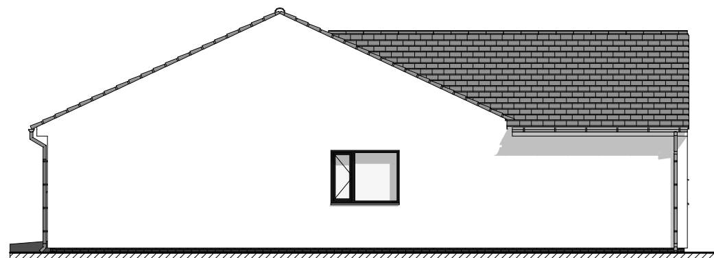
Elewacja zachodnia
