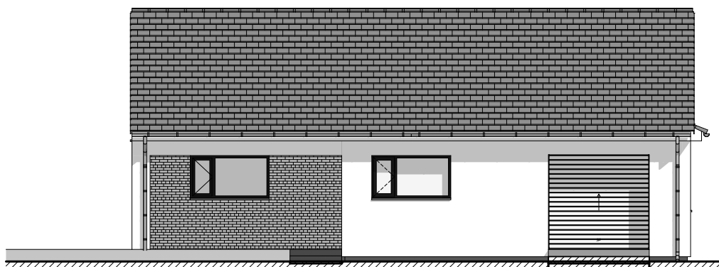
Elewacja frontowa
