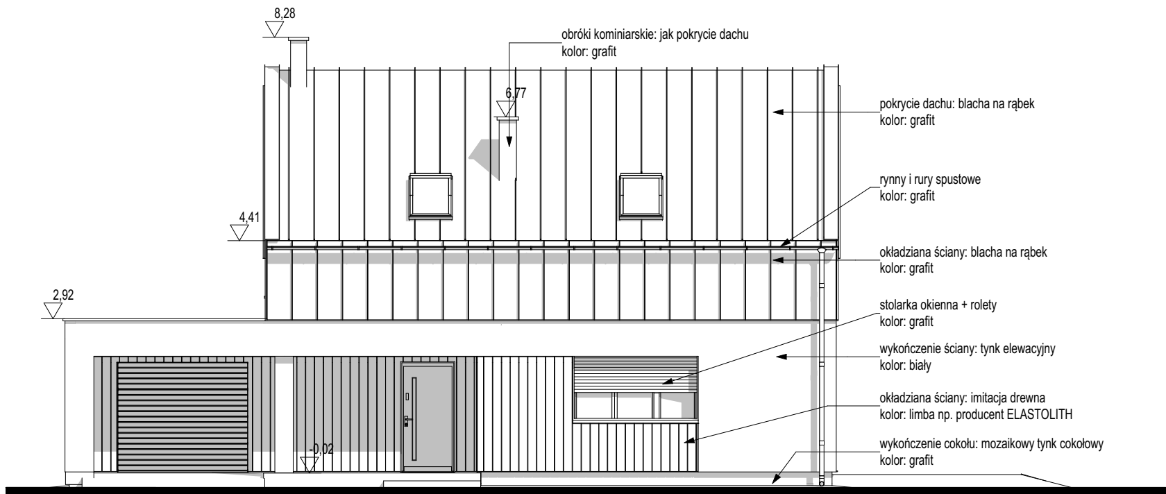
Elewacja frontowa
